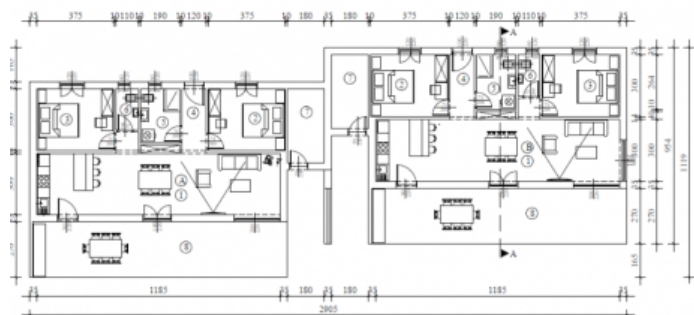
TLOCRT PRIZEMLJA 1:
