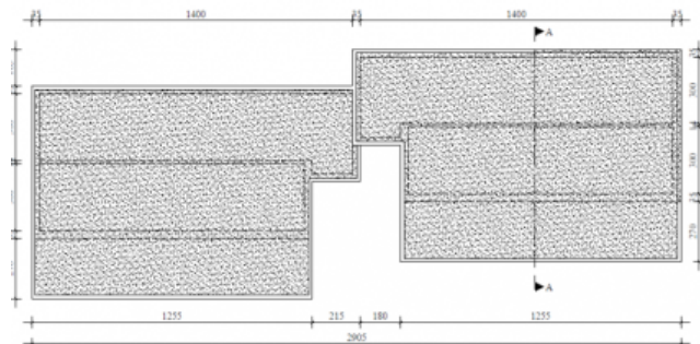
TLOCRT KROVA 1:1
