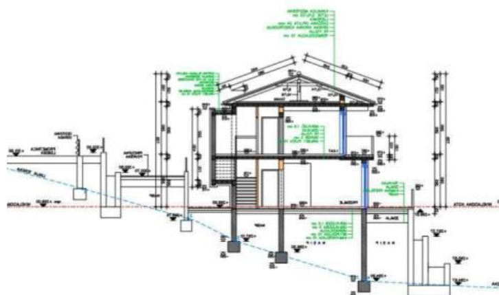
PRESEK M 1:100
