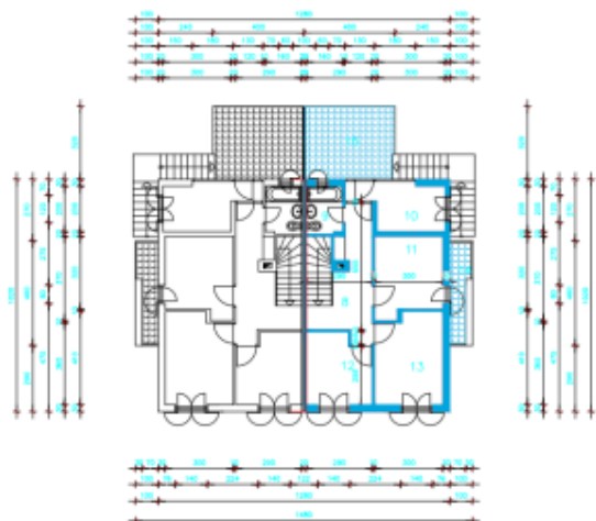
TLOCRT KATI M 1:100
