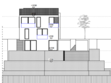
SEVERNO PROČELJE
