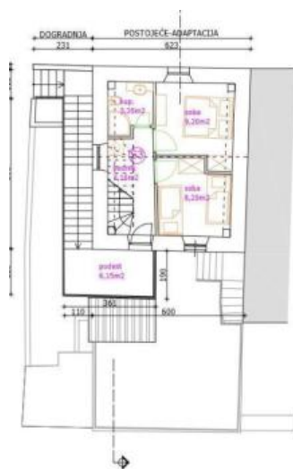
TLOCRT 2. KATA-ADAPTACIJA mj 1:100
