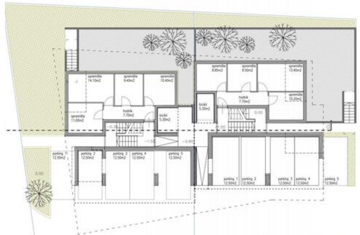
ZGRADA F – tlocrt PODRUMA I PRIZEMLJA
