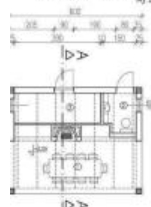
TLOCRT PRIZEMLJA M 1:100
