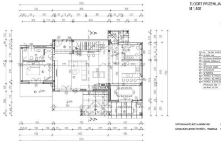
TLOCRT PRIZEMLJA M 1:100
