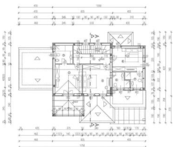
TLOCRT KATA M 1:100
