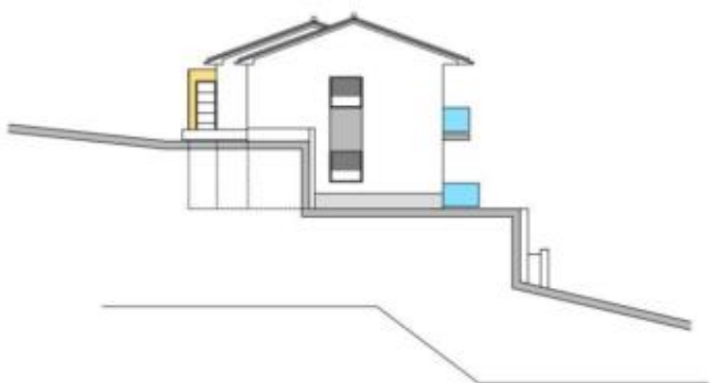
СЕВЕРНА ФАСАДА М1:100
